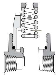
FIGURE 2 – Régulateur miniature, sans équilibre, avec dispositif d'évacuation montré
